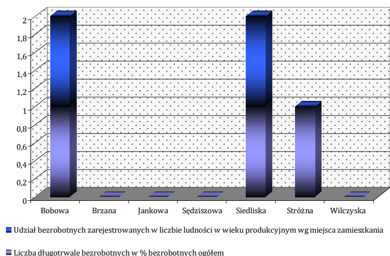
Rysunek 16. Zestawienie wskaźników ze sfery społecznej rynku pracy
